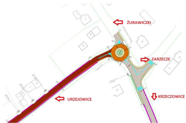
Projektowane rondo na skrzyżowaniu w Żurawiczkach – Kamienia
